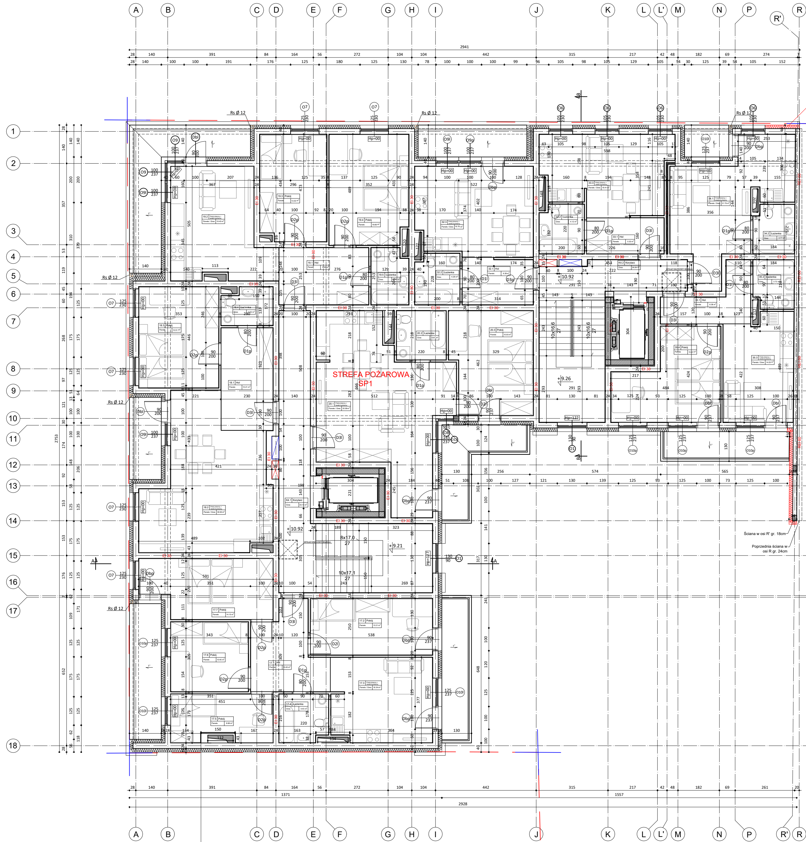
RZUT PODDASZA
